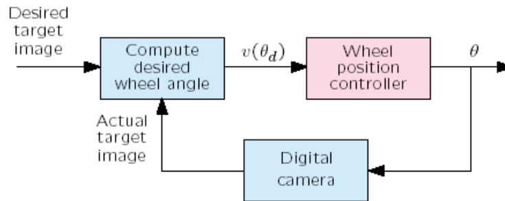
Gambar 1. Navigasi visual dari mobile robot .
